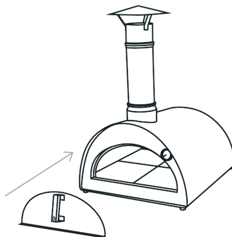
5 - Fit door
